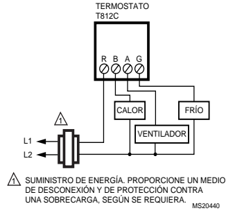
Fig. 7. T812C en sistema de calefacción y enfriamiento.
