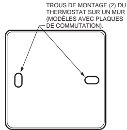
Fig. 3. Emplacement des trous de montage sur les modèles avec plaque de commutation.
