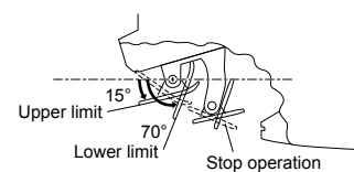
FAN operation
